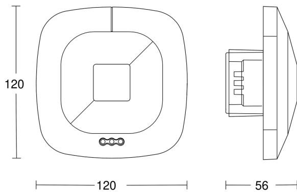
Technische Zeichnungen
