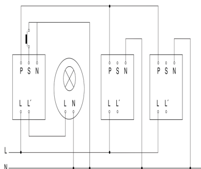
Schaltplan Master
