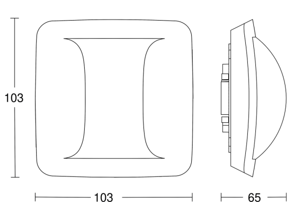
Technische Zeichnungen
