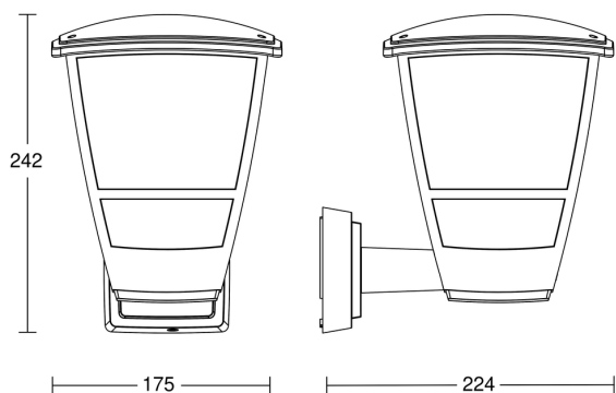
Technische Zeichnungen
