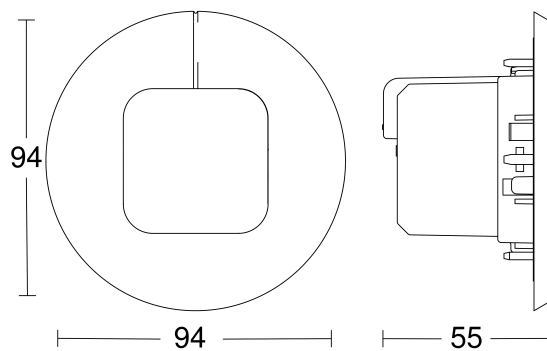
Technische Zeichnung
