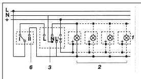
3. Liitäntä vaihtokytkimellä jatkuvaa valaisua ja automaattikäyttöä varten
