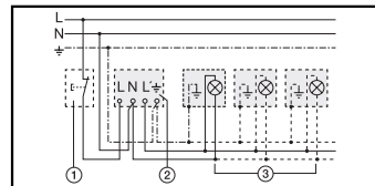
1) Openschakelaar, 2) BLS T, 3) Verbruiker, verlichting
