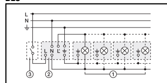
1) Gruppo di lampade, 2) BLS, 3) Interruttore esterno
