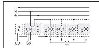
1) Lampengroep, 2) BLS, 3) Externe schakelaar
