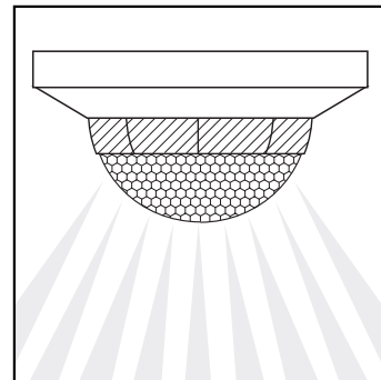
Waagerechte Trennung = Reduzierung der Reichweite
