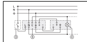
4) Lampe med DIMM elektrodrosselspole, 5) BLS D / BLS DF
