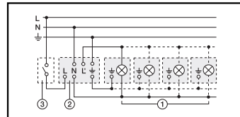
1) Valaisinyhmä, 2) BLS, 3) Erillinen kytkin
