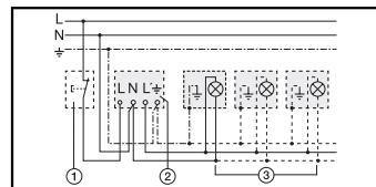
1) Öffnertaster, 2) BLS T, 3) Verbraucher, Beleuchtung
