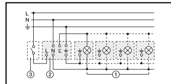
1) Lampegruppe, 2) BLS, 3) Ekstern bryter
