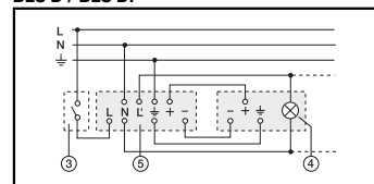
4) Lampada con ballast elettronico DIMM, 5) BLS D / BLS DF
