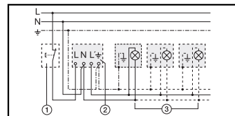
1) Åpnerast, 2) BLS T, 3) Apparat, belysning
