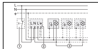
1) Avauspainike 2) BLS T, 3) Sähkölaite, valaistus
